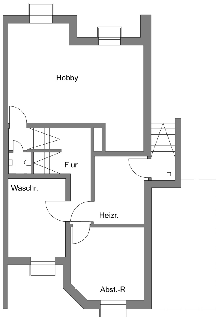
Kellergeschoss
