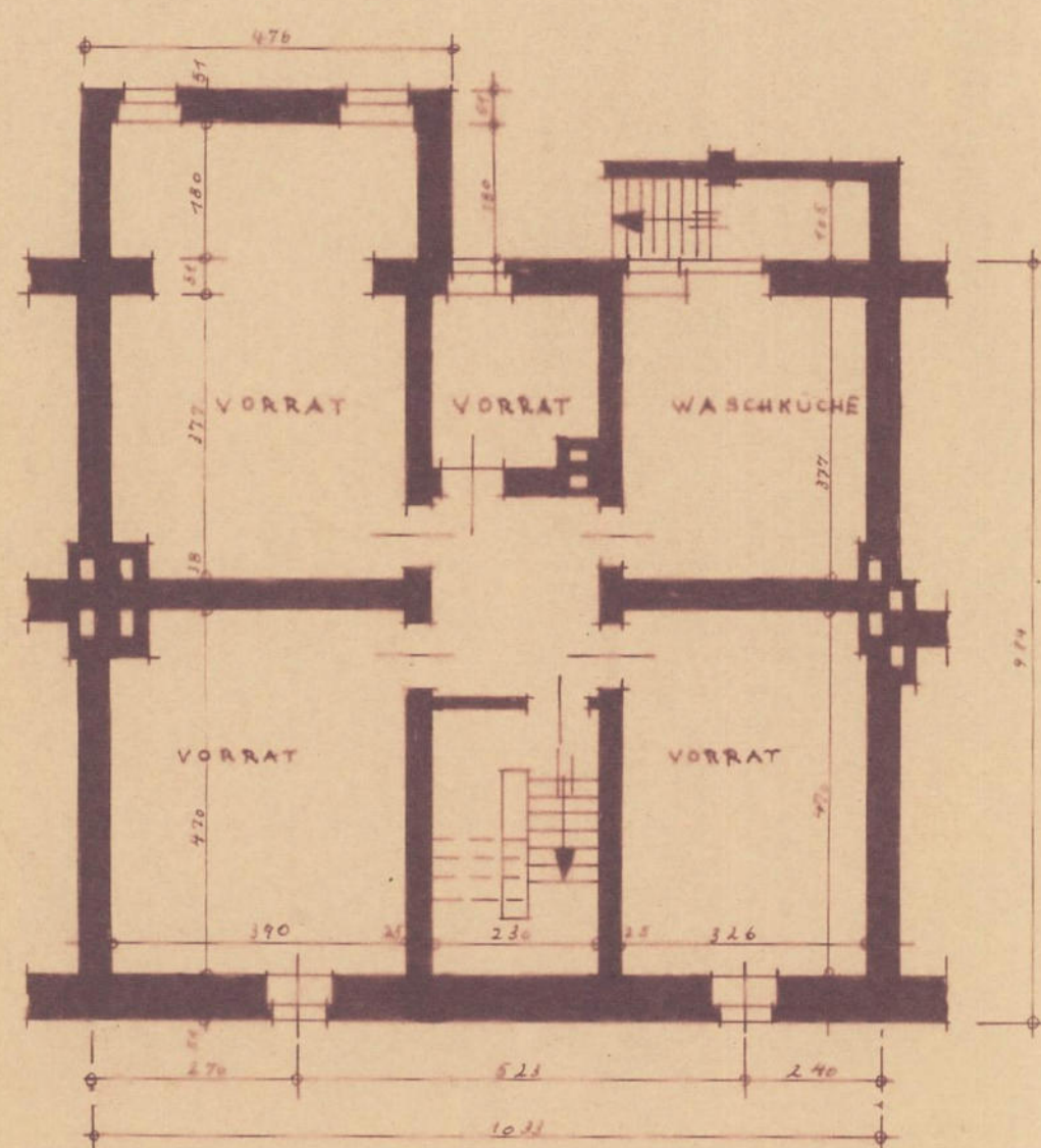
KELLERGECHOSS
