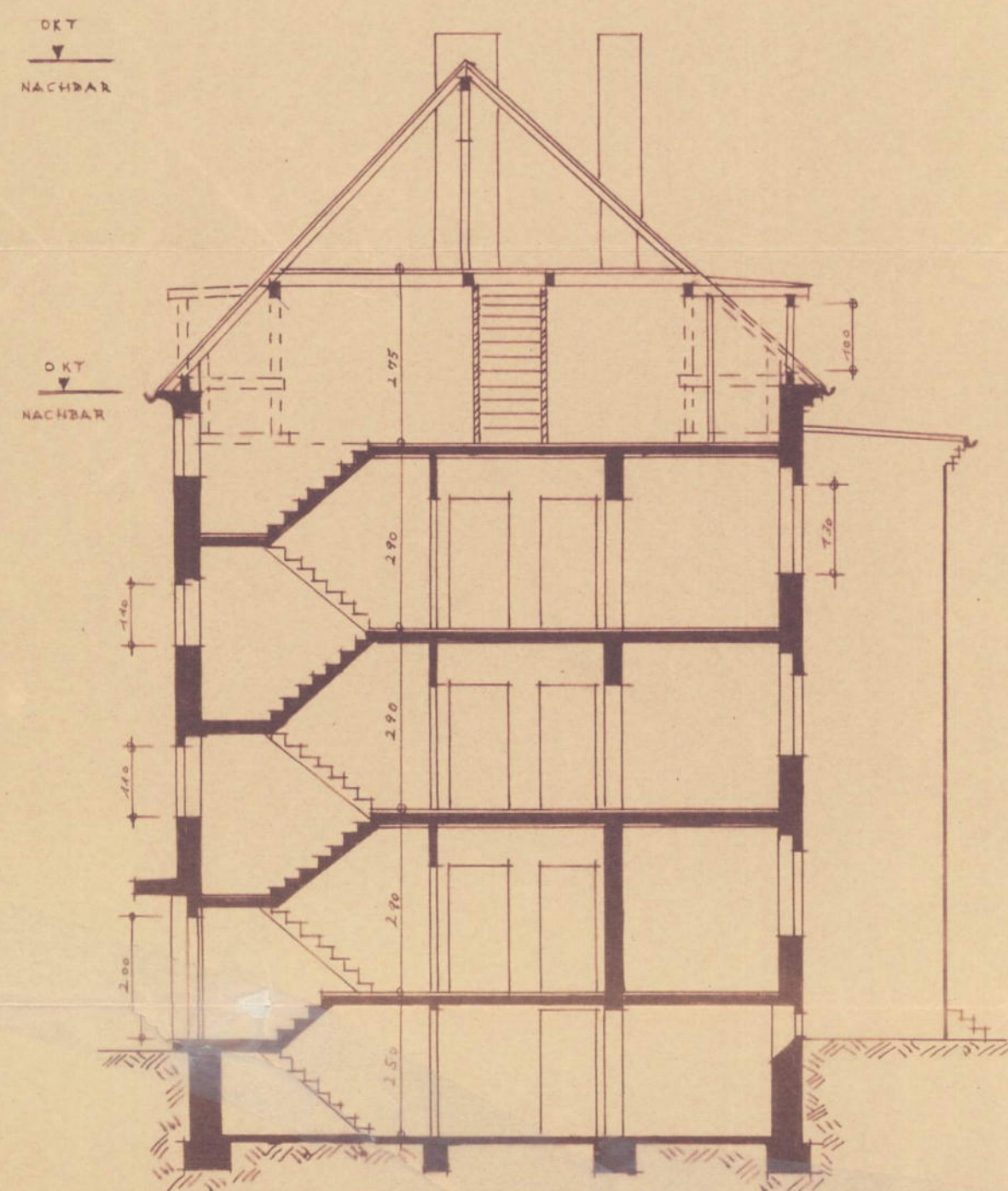
QUERSCHNITT
