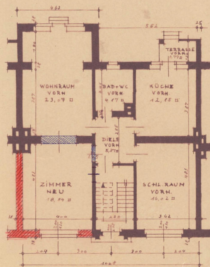
ERDGESCHOSS
