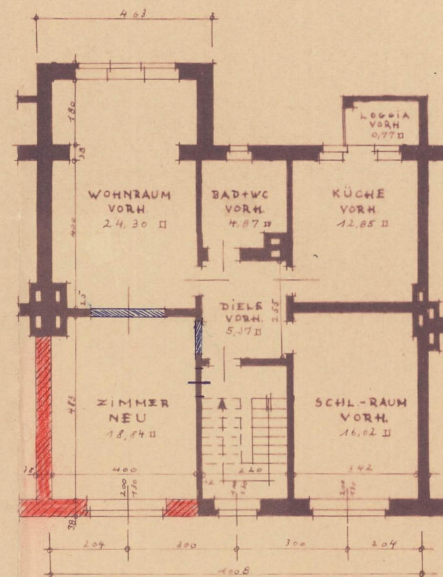
1. OBERGESCHOSS
