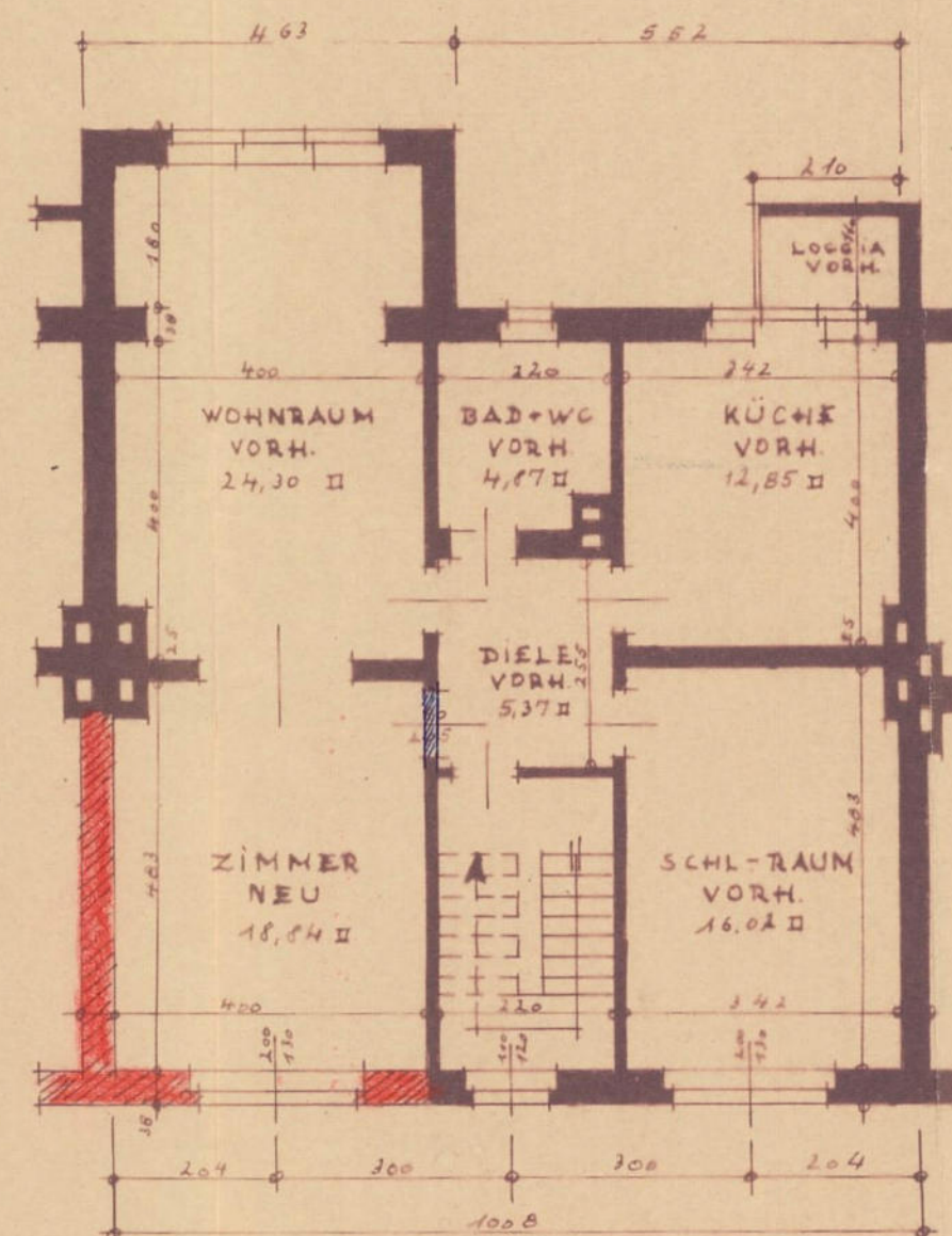
2. OBERGESCHOSS
